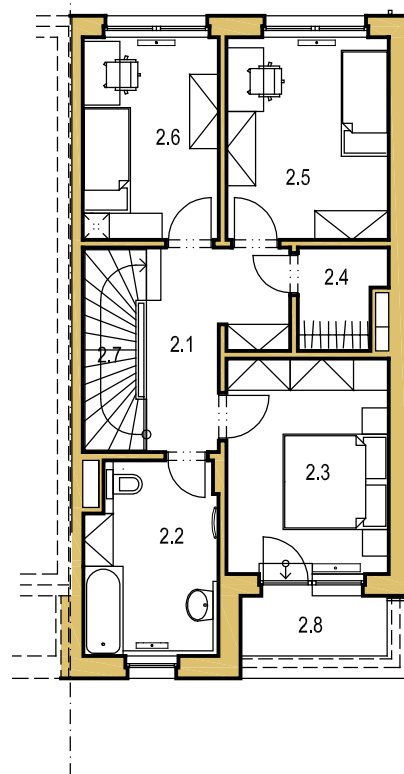
Tabulka místností - 2.NP
