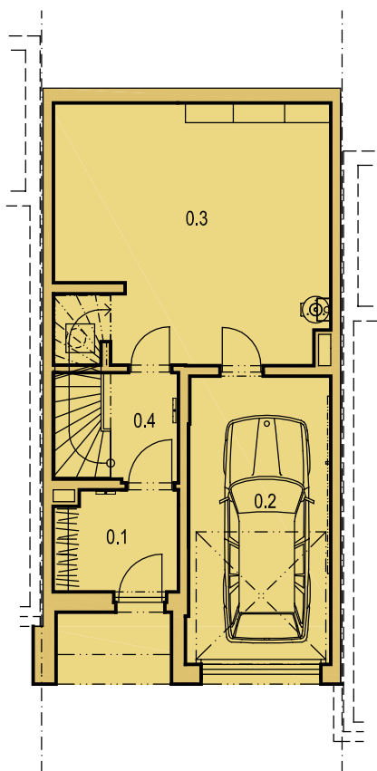
Tabulka místností - 1.PP
