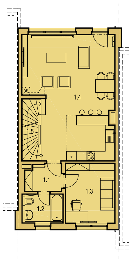
Tabulka místností - 1.NP
