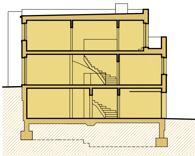
řez domu A-A
